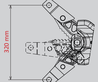
Zugaufsatz ID 2836033
